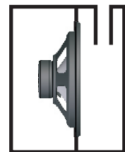
CAIXA BAND-PASS
