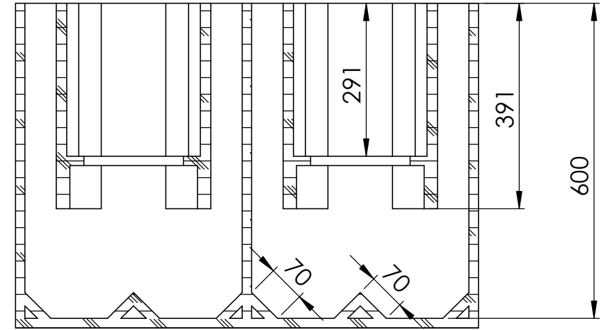
SEÇÃO A-A
